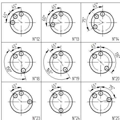
Exemple d'écrous de verrouillage
